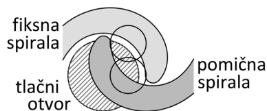
Slika 3.19 Detalj središnjeg dijela spiralnog kompresora s tlačnim otvorom (plavo), fiksnom (crno) i pomičnom spiralom (crveno)
